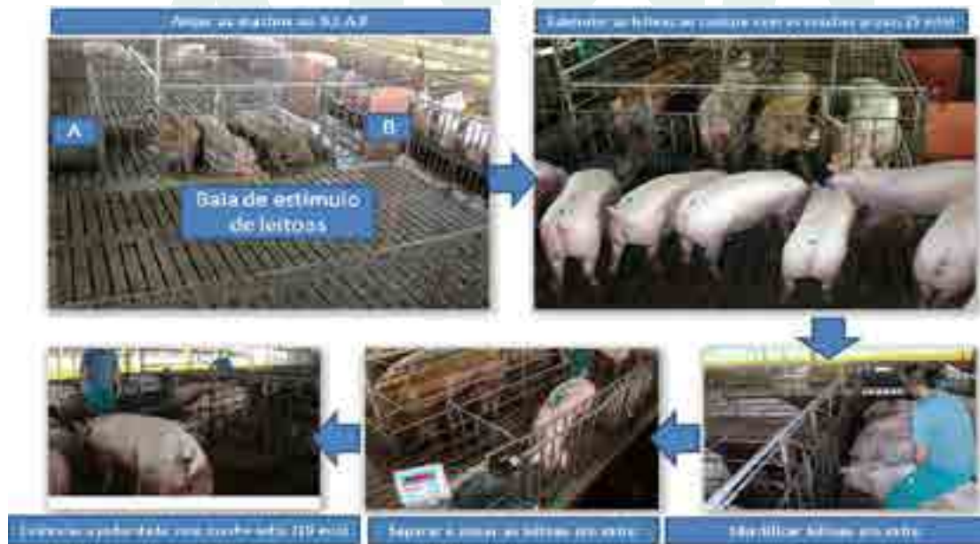
A: Balança B: Cela de retenção de leitoas em estro
