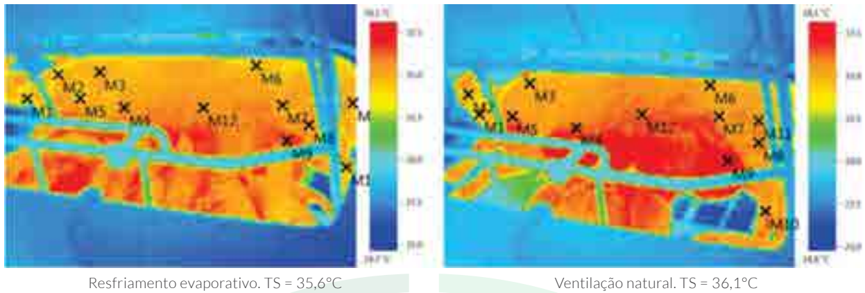
Figura 2 - Imagens termográficas das temperaturas superficiais (TS) de porcas em lactação, no período da tarde (entre 15h e 17h), de acordo com o sistema de ventilação
